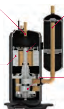
Sprężarka inwerterowa Twin Rotary
